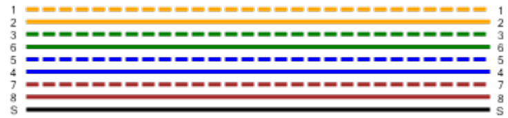
T568B
